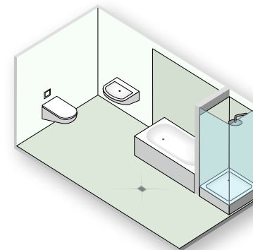
f Häusliches Bad mit Badewanne ohne Brause und mit Duschtasse mit Duschtabtrennung; Bodenablauf im Raum.
