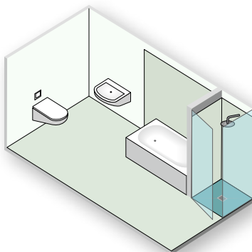
e Häusliches Bad mit Badewanne ohne Brause und mit bodengleicher Dusche mit Duschtabtrennung
